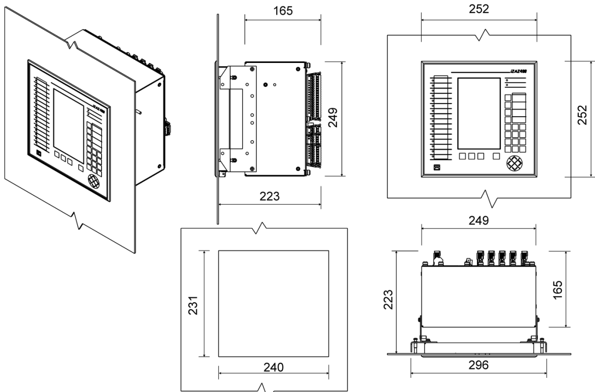
Rys. 13. Wymiary urządzenia iZAZ400 z panelem w wersji P
