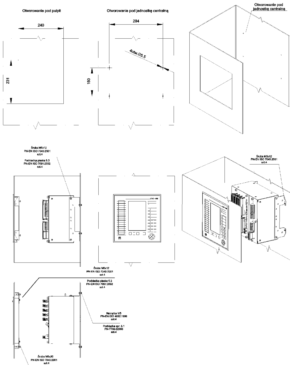
Rys. 17. Sposób montażu urządzenia iZAZ400 – zatablicowy (PAN-P na drzwiach, JP wewnątrz) – wariant B
