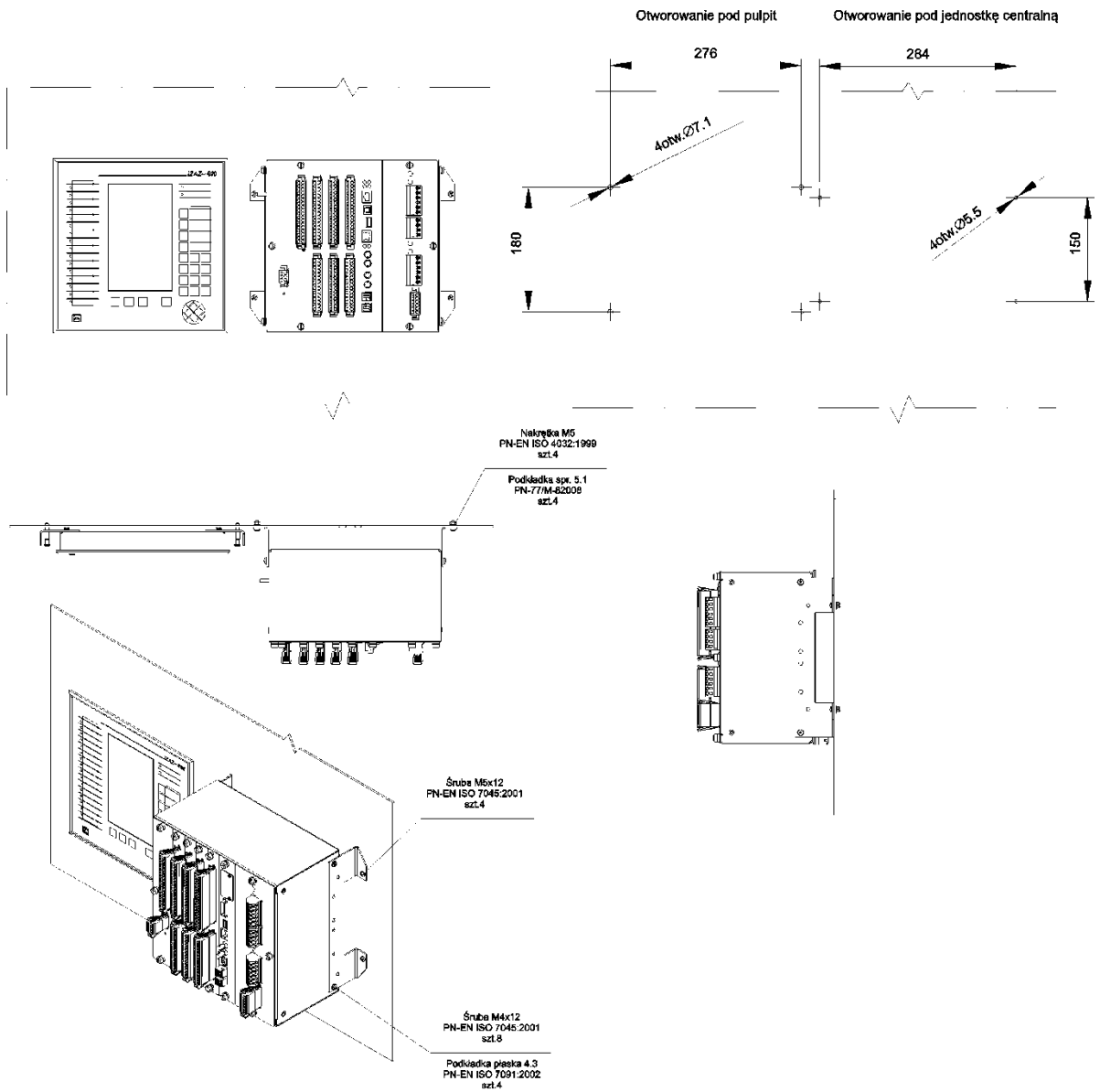
Rys. 19. Sposób montażu urządzenia iZAZ400 – natablicowy – wariant C2
