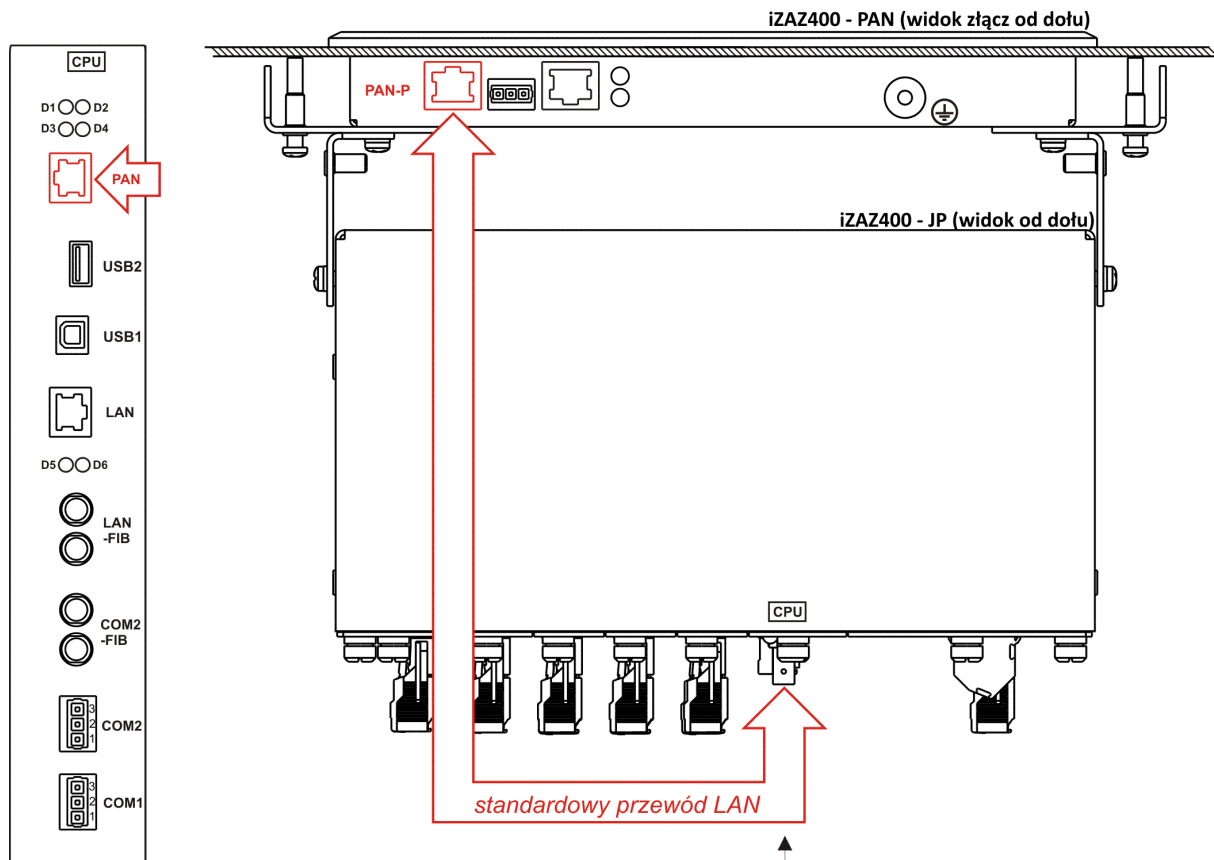
Rys. 27. Sposób podłączenia jednostki podstawowej (JP) i panelu operatora (PAN)
