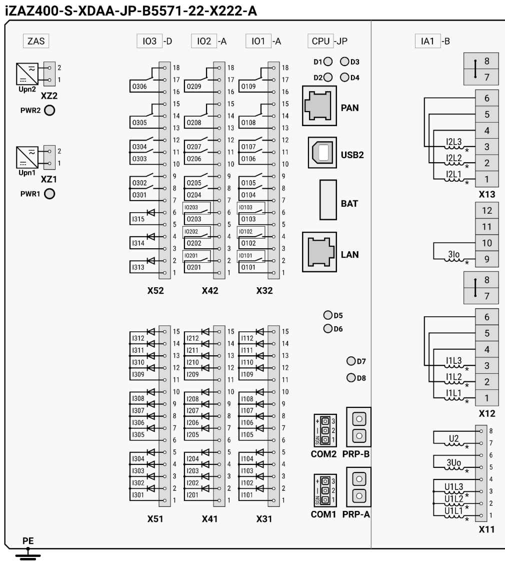
Rys. 1. Schemat połączeń zewnętrznych dla iZAZ400 (przykład dla XDAA)
