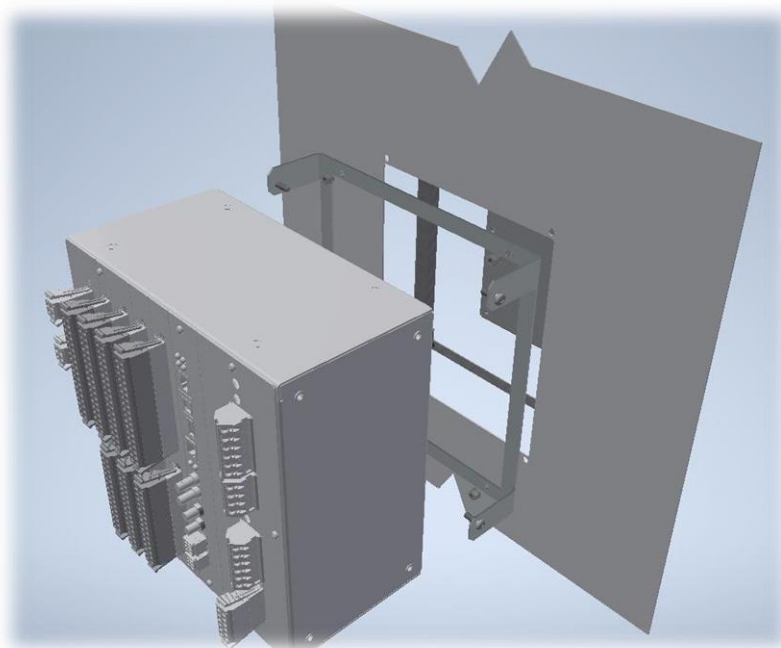
Rys. 24. Sposób montażu urządzenia iZAZ400 – panel wariant S – wizualizacja tył
