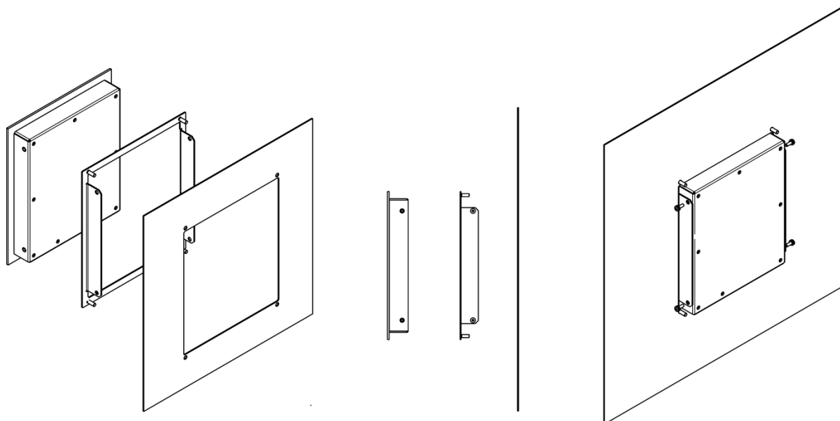
Rys. 20. Sposób montażu urządzenia iAZ400 – panel wariant 2
