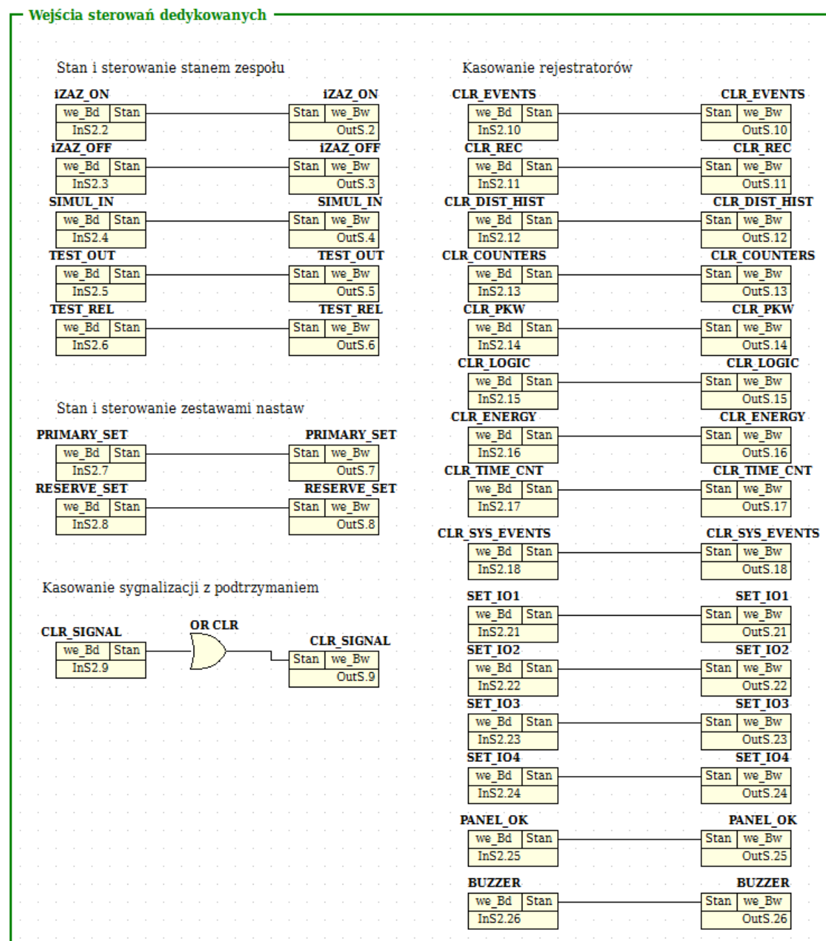
Rys. 12. Arkusz połączeń wejść impulsowych statusów dedykowanych – iZAZ Tools
