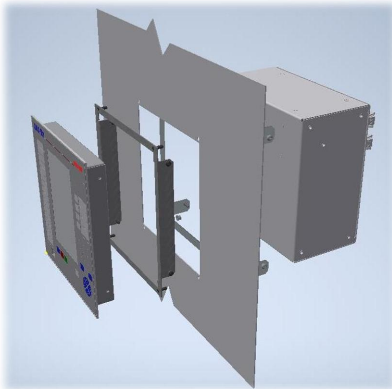
Rys. 23. Sposób montażu urządzenia iZAZ400 – panel wariant S – wizualizacja przód
