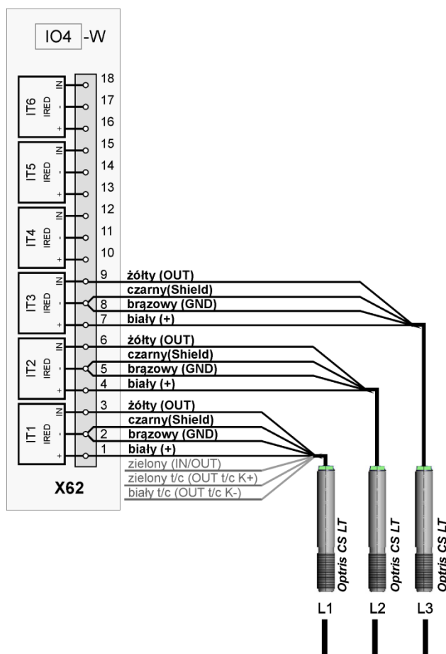
Rys. 6. Sposób podłączenia czujnika temperatury IRED.
