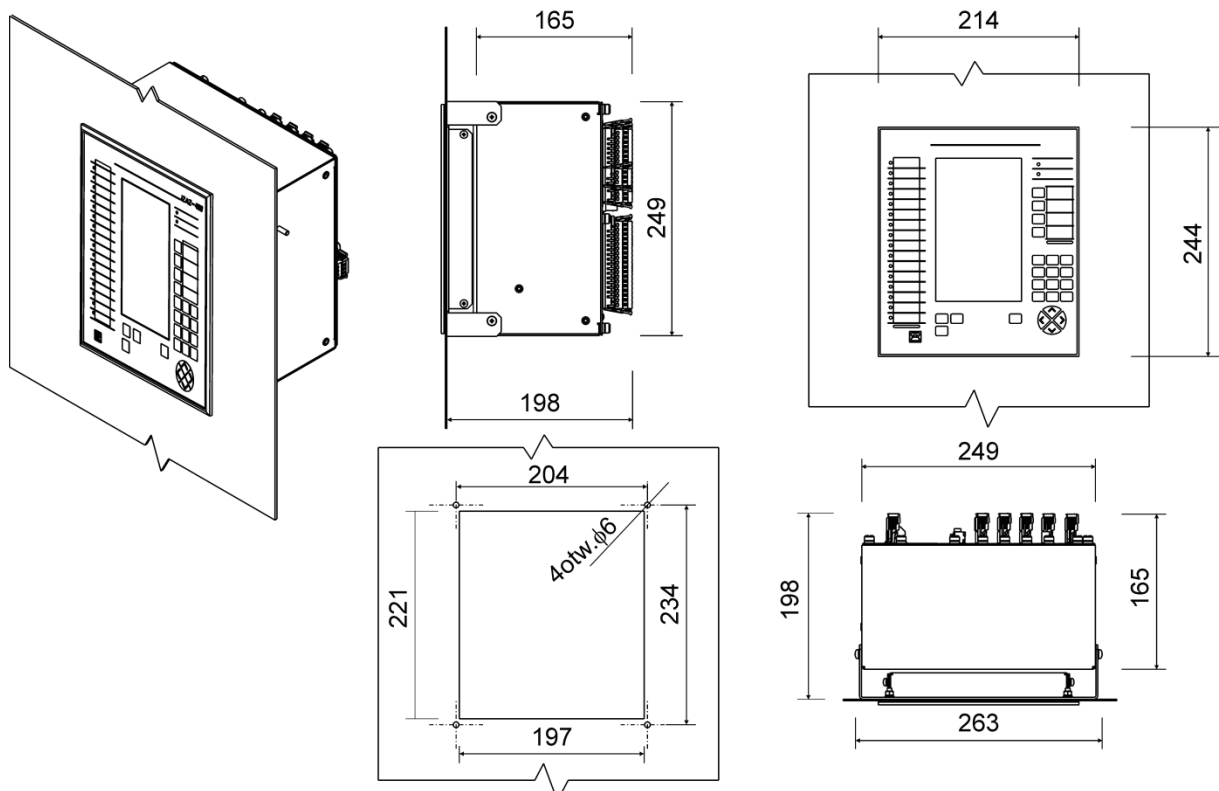
Rys. 14. Wymiary urządzenia iZAZ400 z panelem w wersji S
