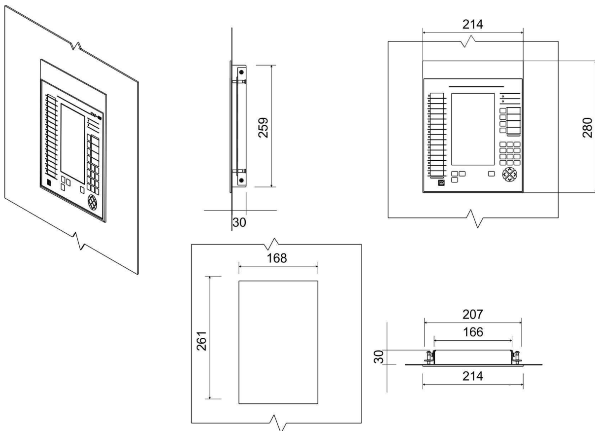
Rys. 25. Sposób montażu urządzenia iZAZ400 – panel wariant M – wymiarowanie
