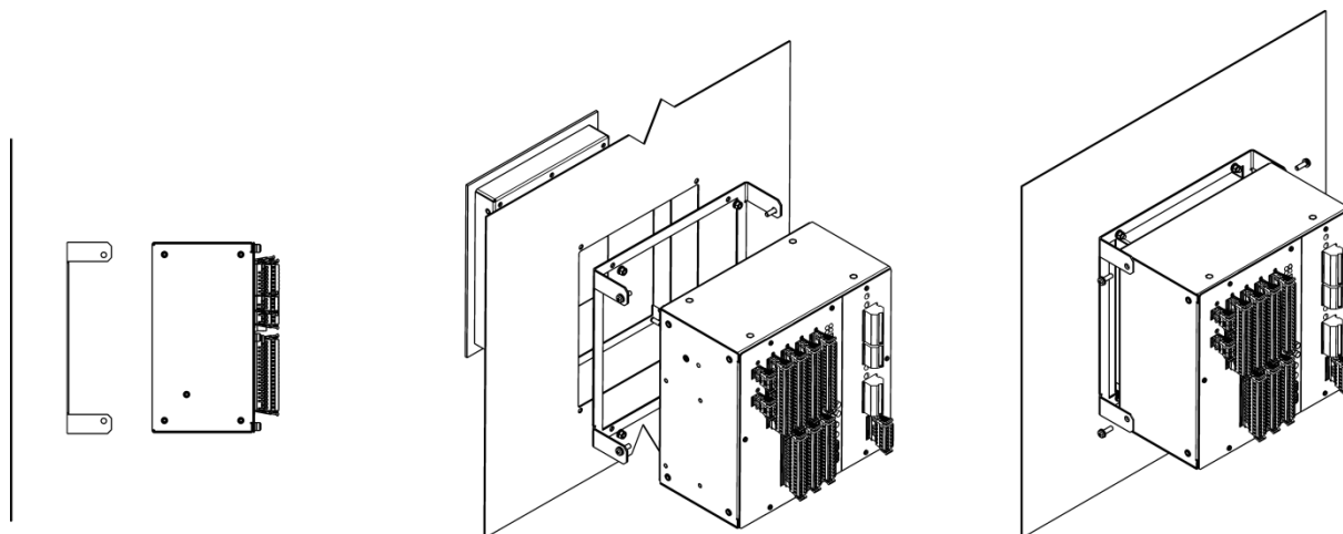
Rys. 21. Sposób montażu urządzenia iAZ400 – panel wariant 2 – jednostka centralna
