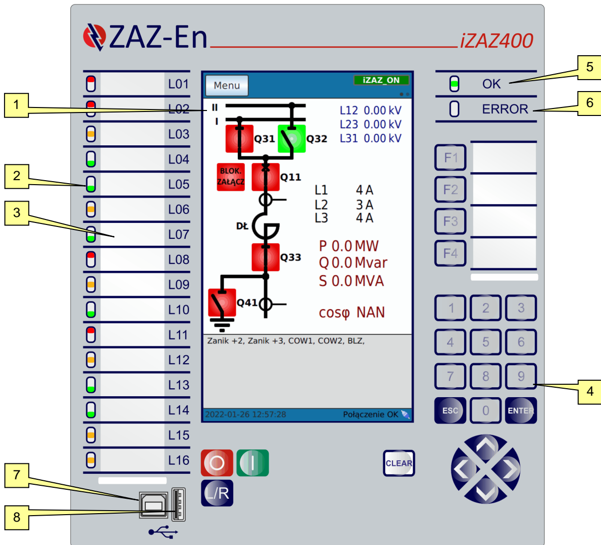
Rys. 29. Płyta czołowa wariantu 2 – panel operatora iZAZ400
