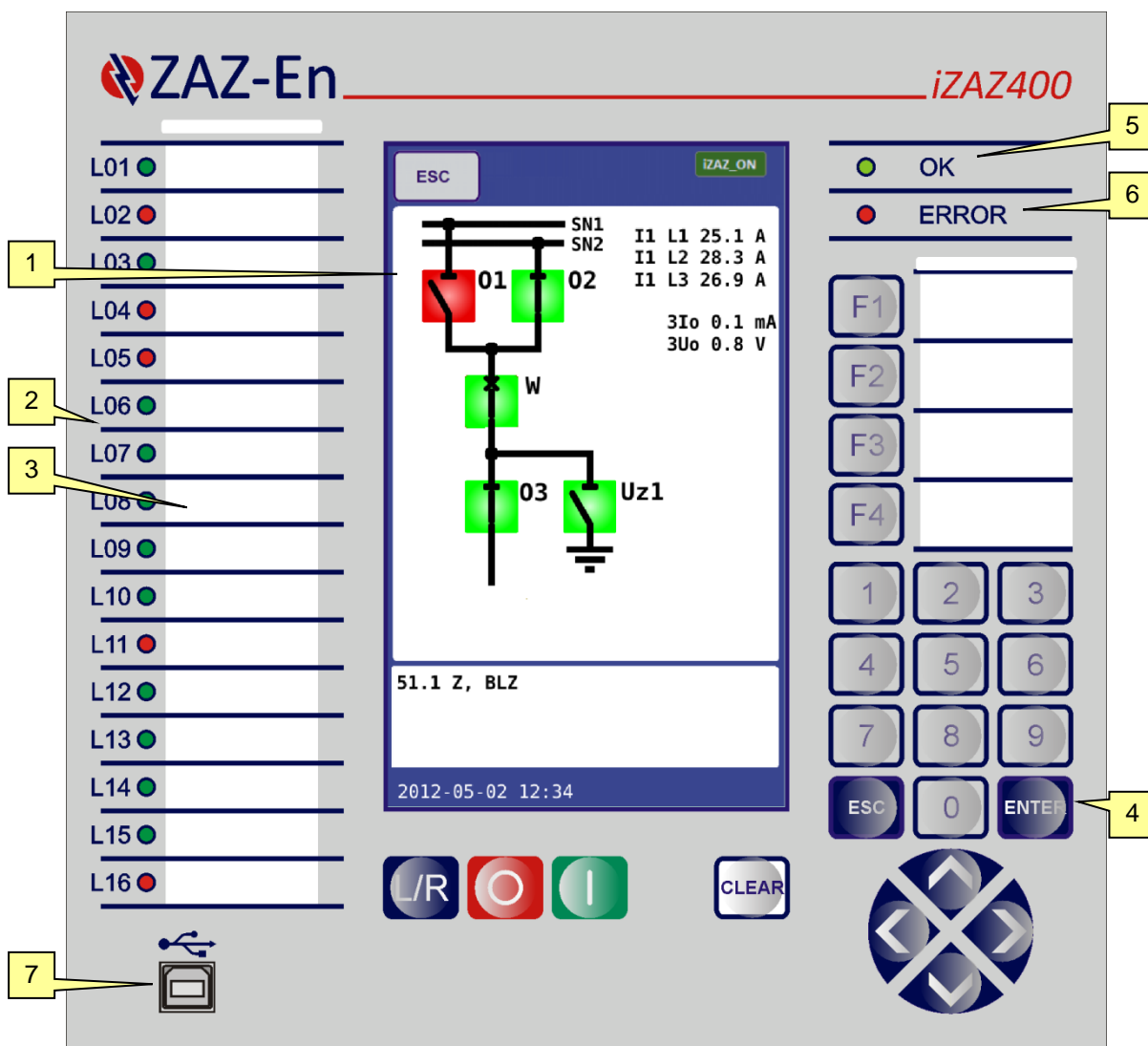
Rys. 28. Płyta czołowa wariantu 1 – panel operatora iZAZ400
