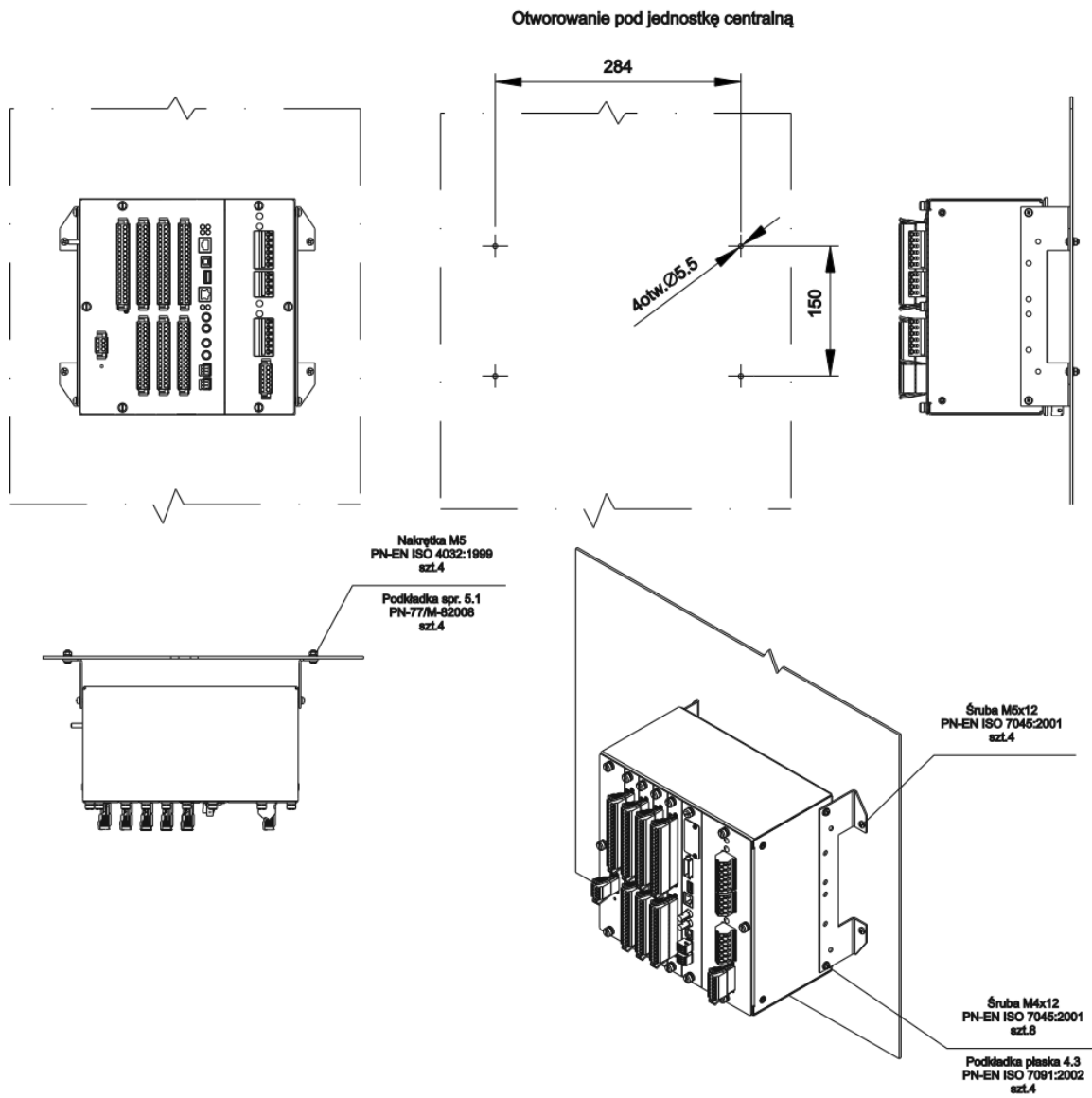
Rys. 26. Sposób montażu urządzenia iZAZ400 – jednostka centralna dla wersji M panelu
