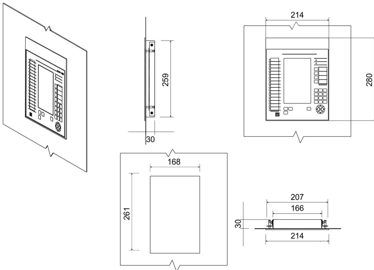
Rys. 15. Wymiary urządzenia iZAZ400 z panelem w wersji M
