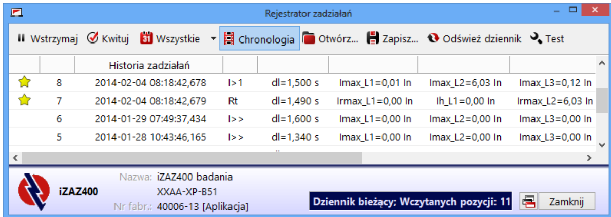
Rys. 10. iZAZ Tools – przykładowe okno rejestratora zadziałań
