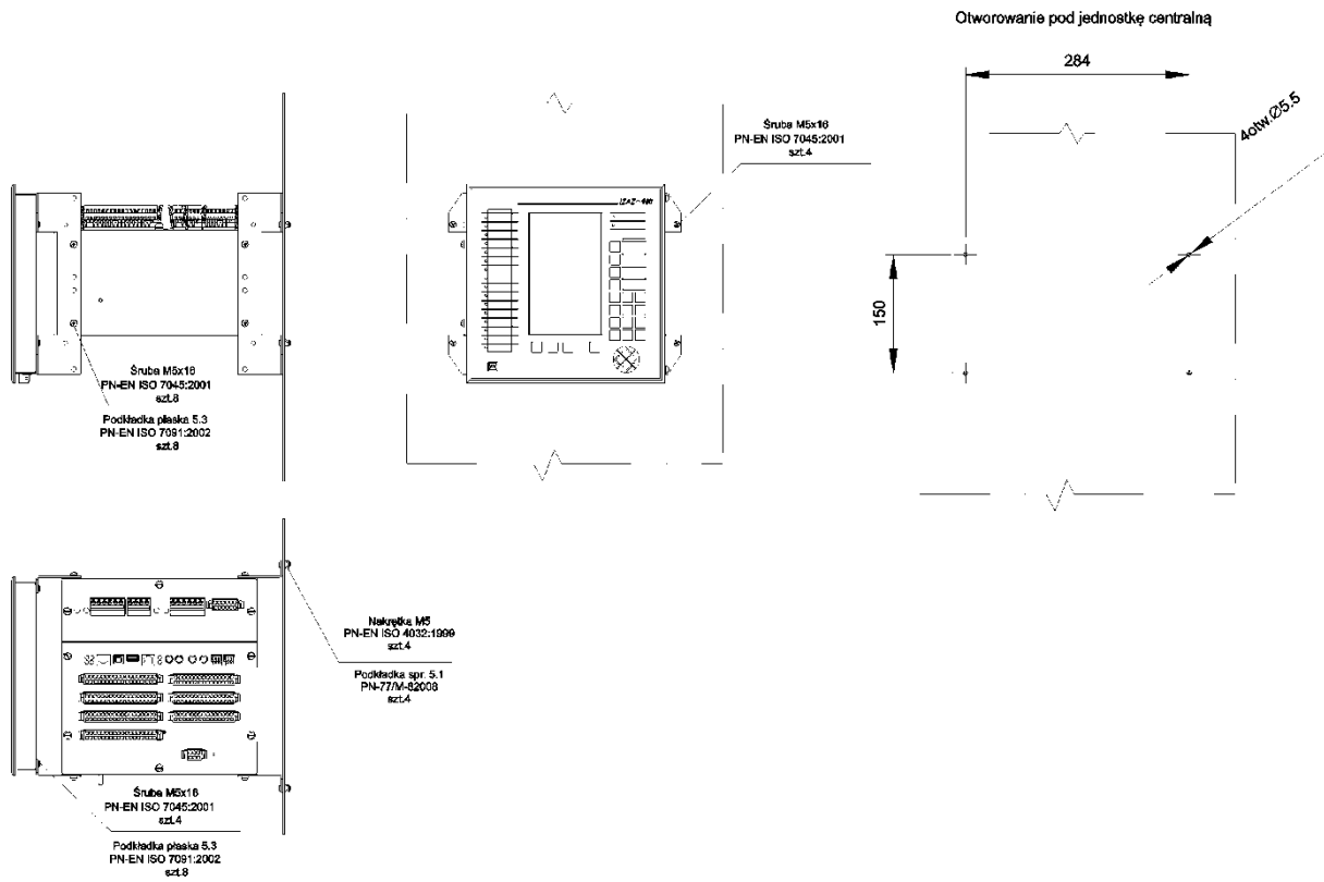
Rys. 18. Sposób montażu urządzenia iZAZ400 – natablicowy – wariant C1
